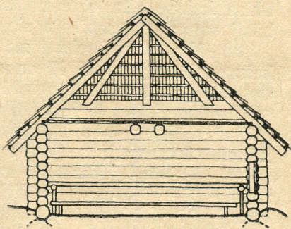
Lõige GH
