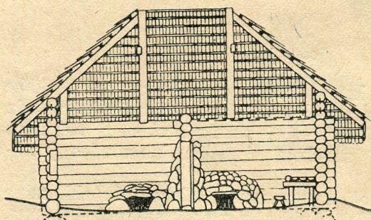
Lõige ABCD
