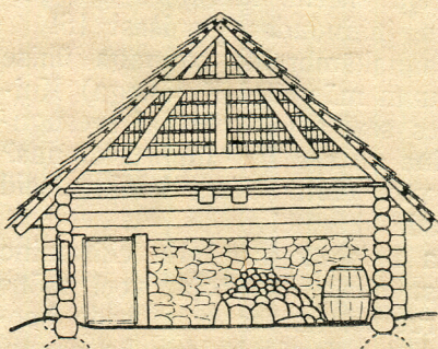
Lõige EF
