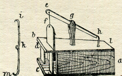
Joon. 8. Kastikujuline lõks.
