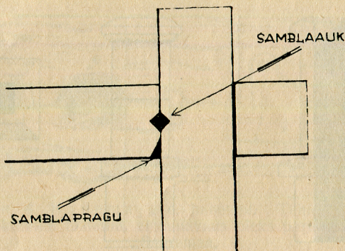
Joon. 2. Eelmine nurk kokkupandult. Nooltega on näidatud samblaauku ja samblaprao asend pealtvaates.
