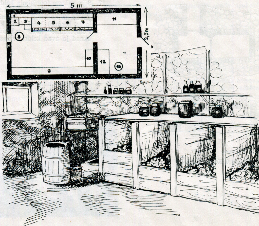
Joonis 8. Keldri sisustuse skeem ja sisevaade. Tartu.
