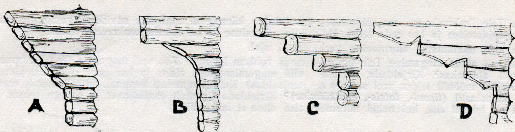
Joon. 9. Aida kandenurki: A — Karula, B — Kihelkonna, C — Kuusalu, D — Nissi (siselõigetega).
