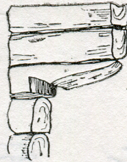
Joon. 8. Aida kande- nurk. Mustjala.
