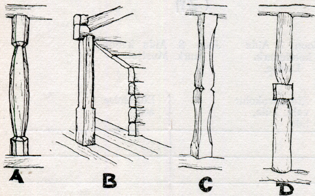
Joon. 10. Aida räästaaluseid kandeposte. A. Halliste, B — Häädemeeste, C — Hageri, D — Halliste
