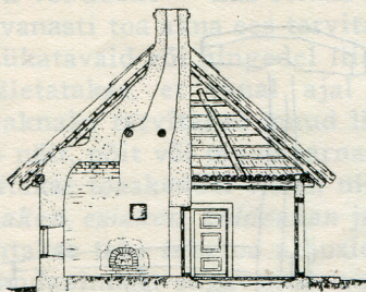
Lõige AB.
