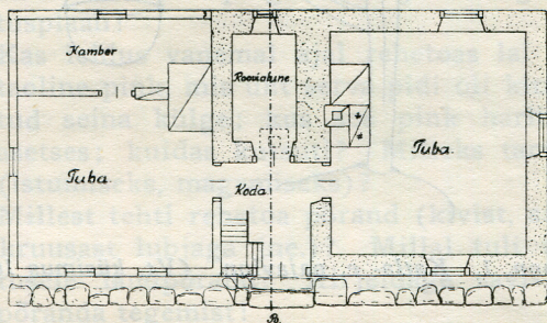
Joon. 2. Roovialuse põhiplaan ja läbilõige. Saaremaal. (Vt. küsimus 22.).
